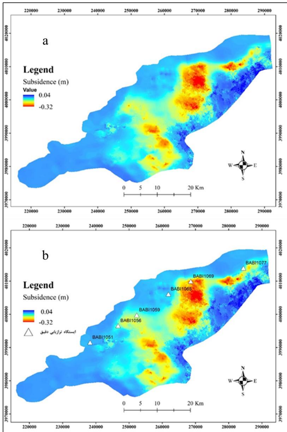
شکل ۵. (a) نقشه پهنه‌بندی نهایی فرونشست زمین در آبخوان دامغان با بیشینه نرخ حدود ۳۲ سانتی‌متر؛ (b) مقایسه نرخ فرونشست سالانه در ایستگاه BABI ۱۰۶۹ بین داده‌های InSAR و ترازبایی دقیق Fig. 5. a) Final land subsidence zoning map of the Damghan plain with a maximum rate of approximately 32 cm; b) Comparison of annual subsidence rates at station 1069BABI based on InSAR and precise leveling data.
